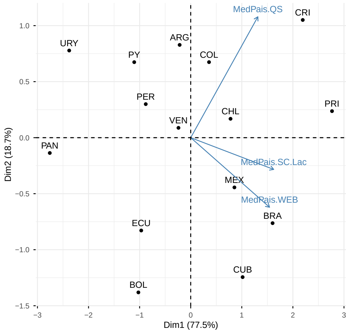
PCA – Biplot
